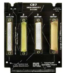
CB7 HD62, HD78 (Item 737)
