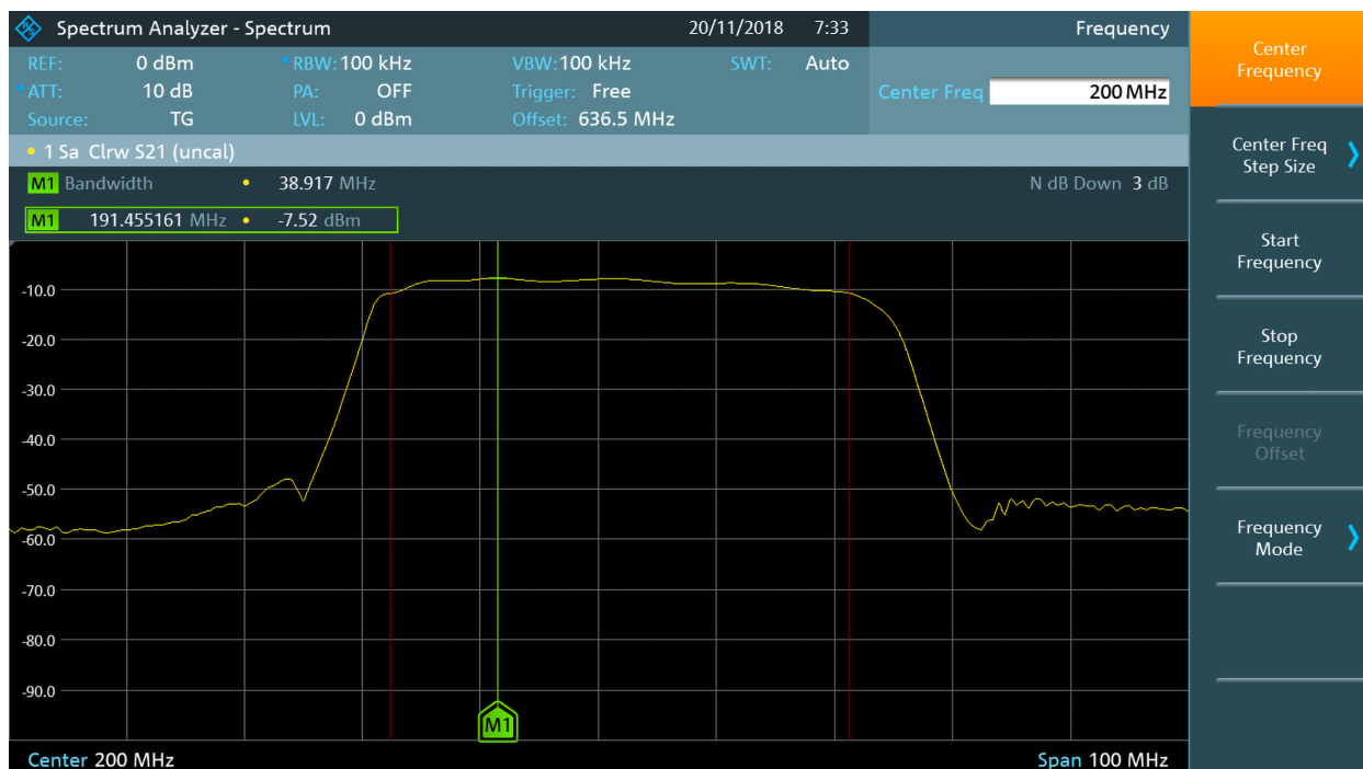
R&S®FPC1500: der Mitlaufgenerator analysiert eine Signalkette mit Mischern, Filtern und Verstärkern
