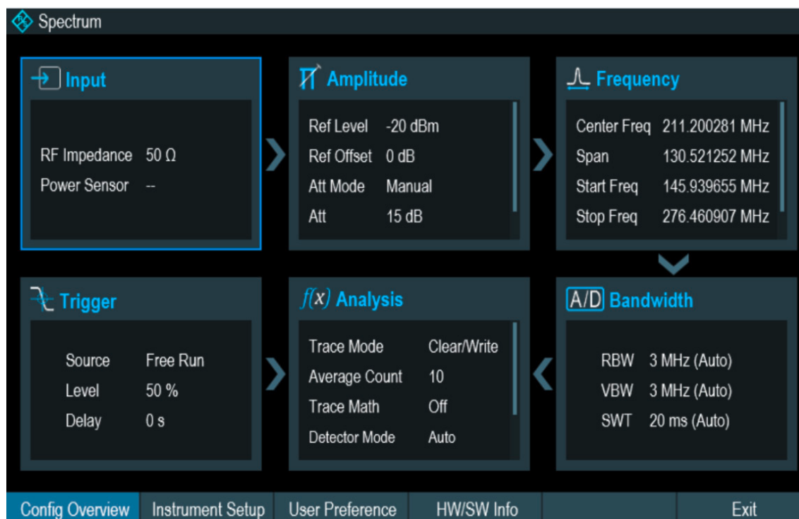
Konfigurations- übersicht
