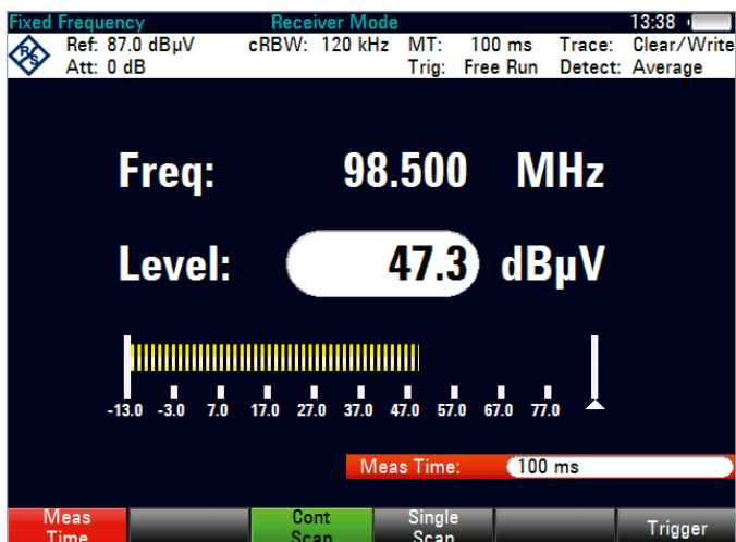
EMV-Precompliance-Messung auf einer festen Frequenz mit einstellbarer Messzeit
