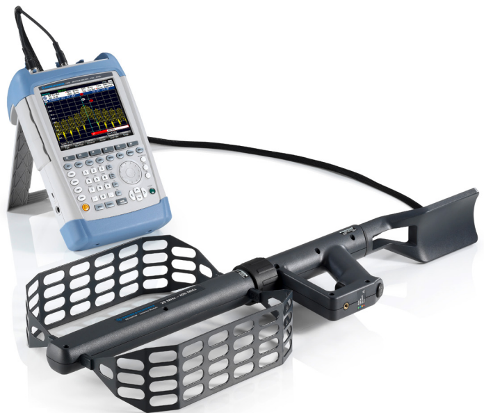
R&S®FSH mit R&S®HE400 Antenne
