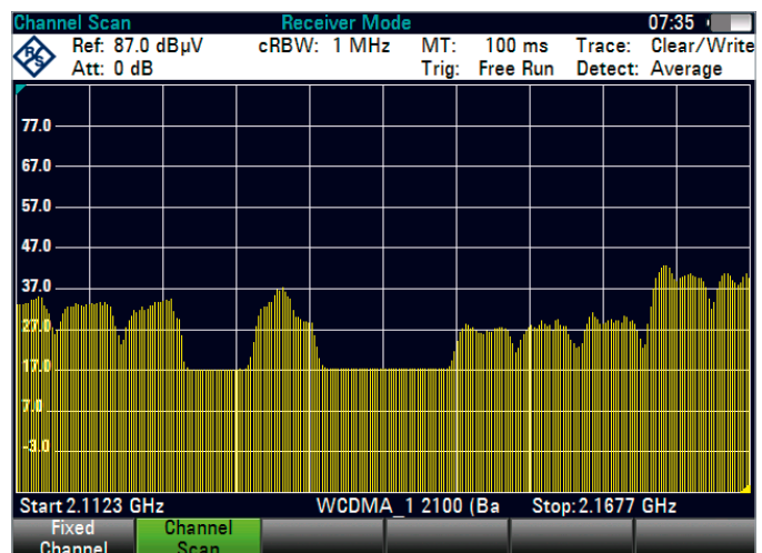
Kanal-Scan eines 3GPP-WCDMA-Frequenzbandes
