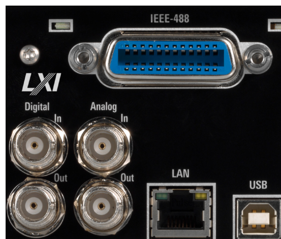
Alle Fernsteueranschlüsse stehen an der Geräterückseite zur Verfügung (Beispiel: R&S®NPA501-G mit IEEE-488-Schnittstelle).
