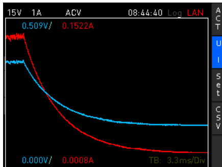
Inrush-Funktion
