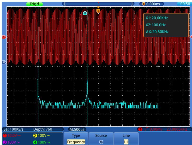
Bild 0-13 Frequenz- Cursormessung im FFT-Modus
