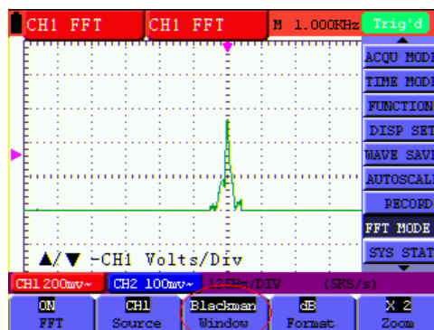
Abbildung 57: Blackman window
