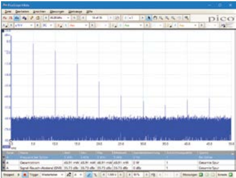
Oszilloskopmodus
