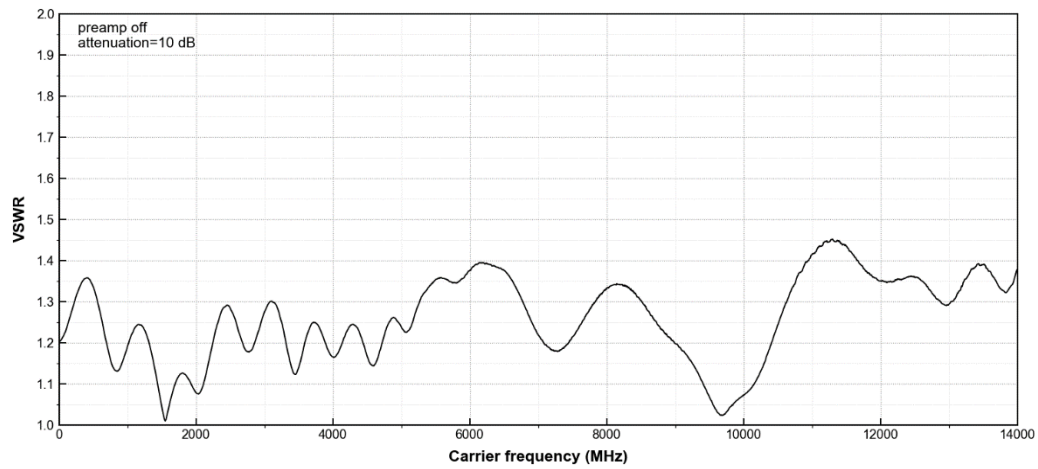
VSWR
