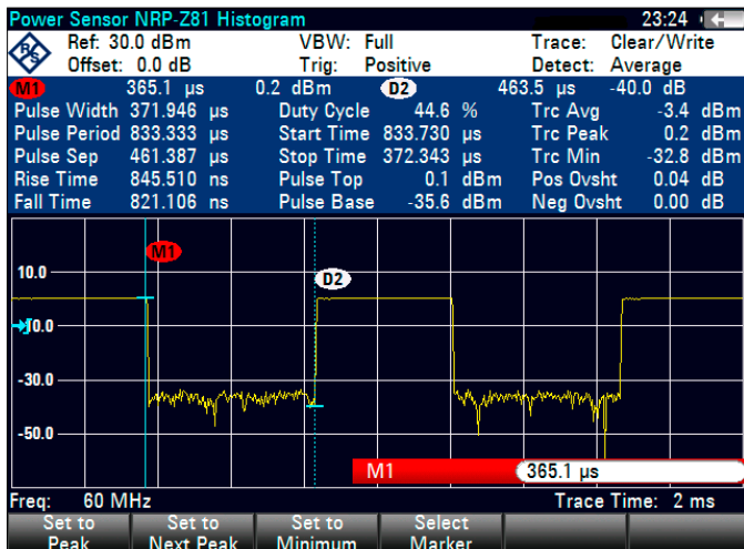
Pulsanalyse mit R&S®ZVH-K29 und dem R&S®NRP-Z81 Breitband-Leistungsmesskopf
