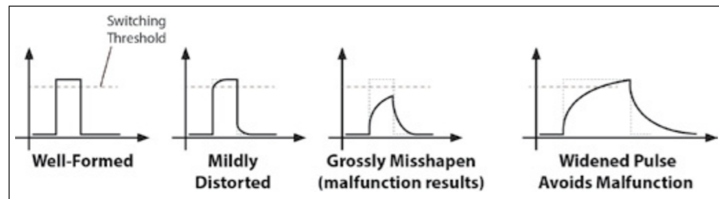
◀ Bild 2: Durch Ausgangsimpedanz und „natürliche“ Kabelkapazität verzerrte Testimpulse (Impulse 2 und 3) können zu Fehlfunktionen führen (Impuls 3), wenn der Prüfpuls nicht eingestellt wird (Impuls 4).
